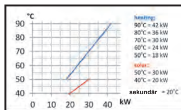
13744 V4A-Heizungssolarwärmetauscher D-SHWT 18 / 35 mit Schlauchmontageset NW 50
